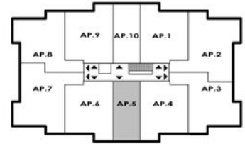
ETAJ II Apartment 5 - garsoniera 1 camera Suprafata Construita = 47.15 m 2 Suprafata Utila = 34.80 m 2 Suprafata terasa = 6.10 m 2
