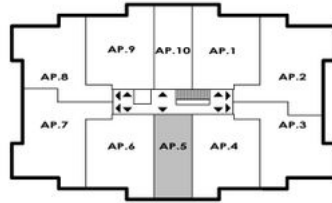
ETAJ I Apartment 5 - garsoniera 1 camera Suprafata Construita = 47.15 m 2 Suprafata Utila = 34.80 m 2 Suprafata terasa = 6.10 m 2
